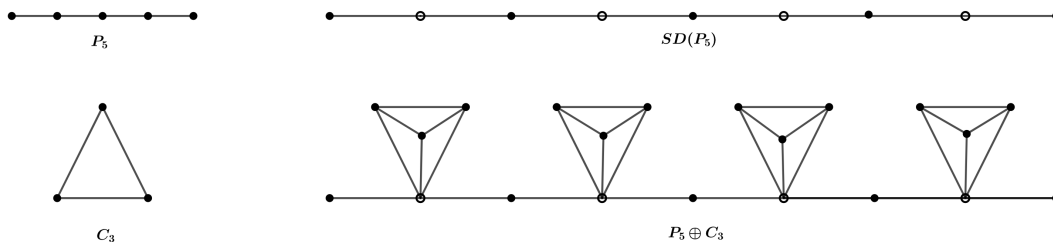
Figure 6. Subdivision - edge corona
